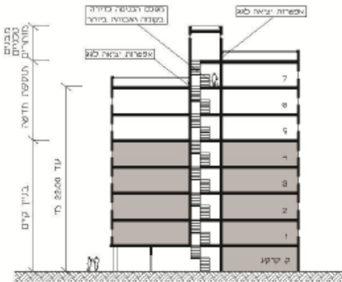
תרשים 3.8.30.4 - תוספת לבניין קיים שאינו גבוה
