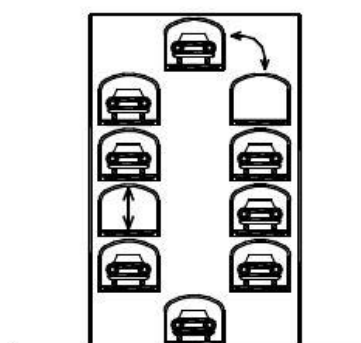
תרשים 10: חניה נעה בסבב אנכי
