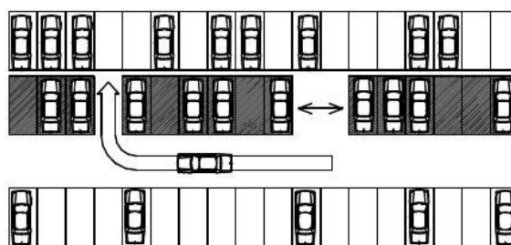
תרשים 3: לוחות חניה זחיתים רוחביים
